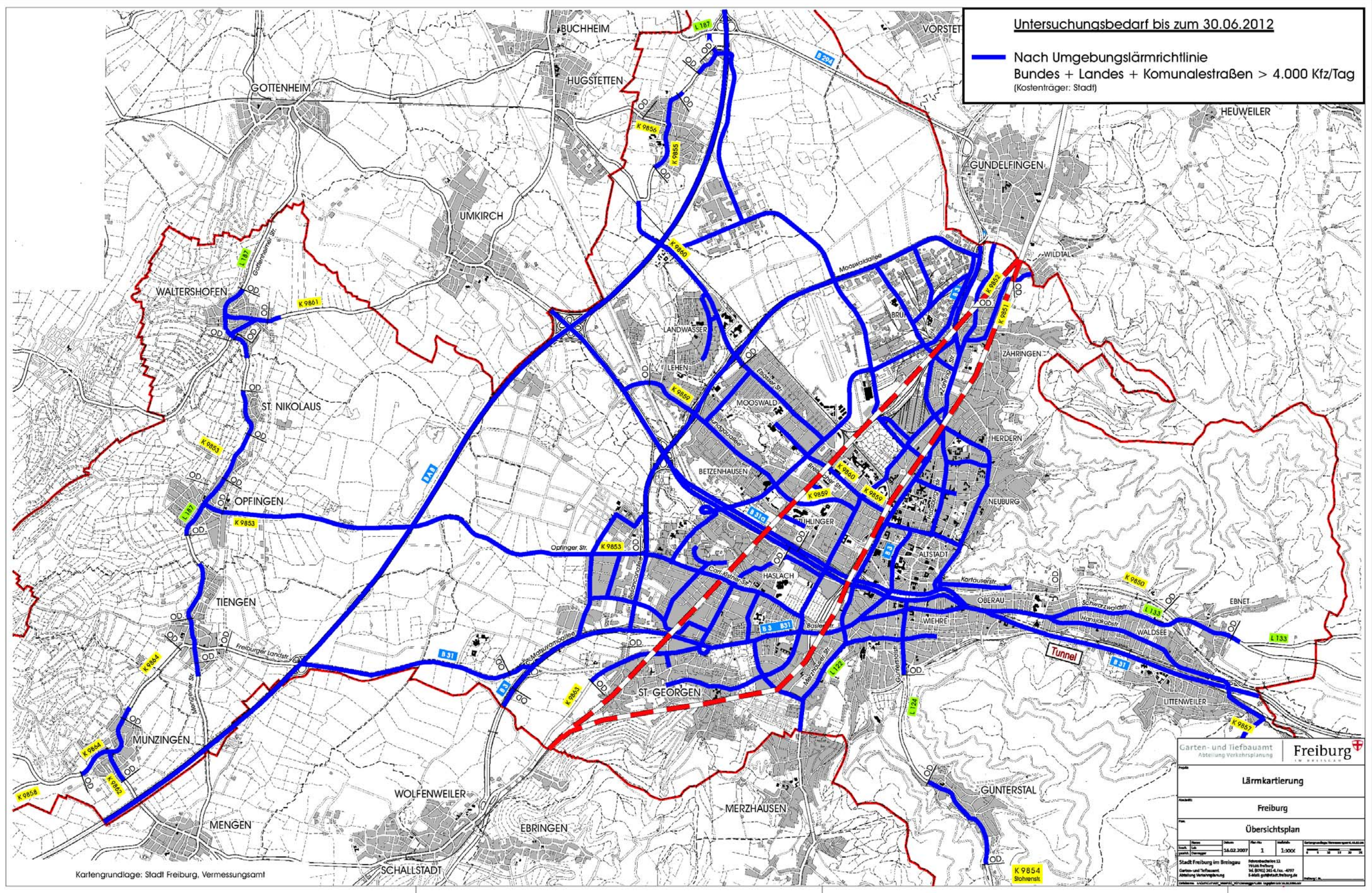
"Umgebungslärmrichtlinien"-Lärmkartierung Stufe 2
