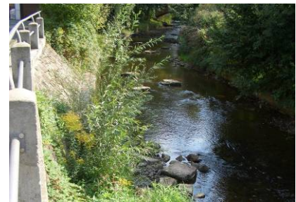
struktureicher Böschungfuß auf engem Raum (Losse, Kassel)
